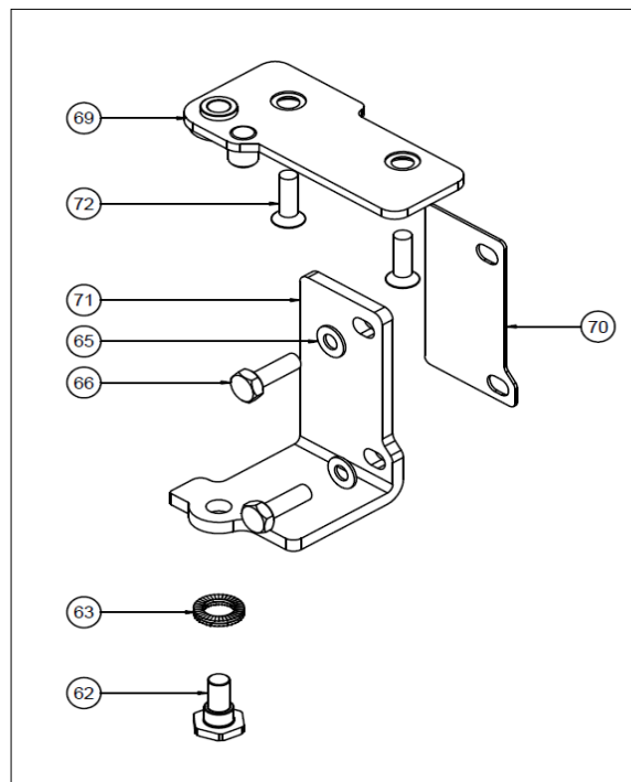
Door Bottom Hinge Assy
